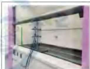
面风速试验 3
